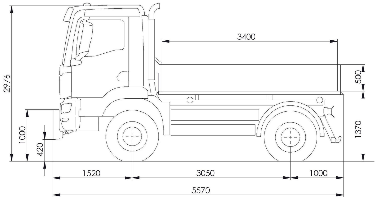
Abbildung 6-1: Maße mit Bereifung v/h: Continental 385/55R22.5 HDC
