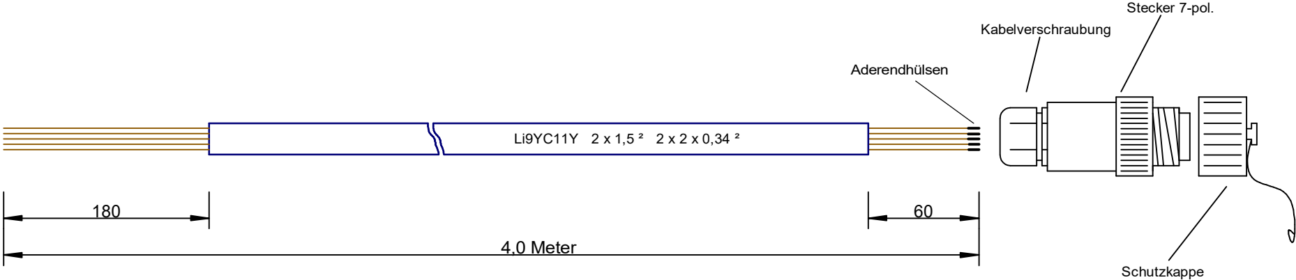
Pin Belegung
